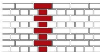
Крестовая. Тип II
