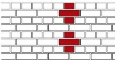
Крестовая. Тип I
