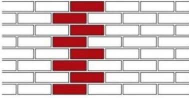
Ложковая в полкирпича
