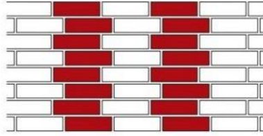
Ложковая в четверть кирпича
